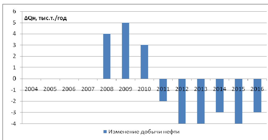
Рис. 67. Изменение добычи нефти в результате проведения ГРП
